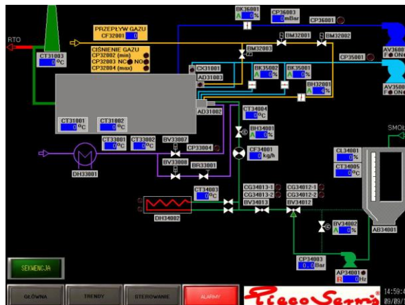
Panel dotykowy z wizualizacją (HMI)
