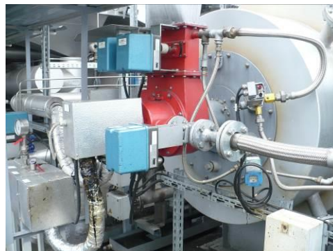
Palnik gazowo-smołowy z zapalarką i nadzorem płomienia
