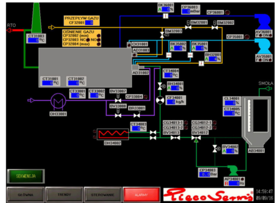
Panel dotykowy z wizualizacją (HMI)
